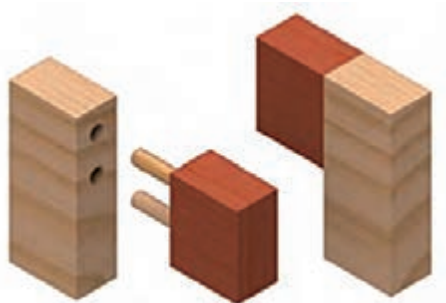
شکل ۲۶- اتصال دوبل
