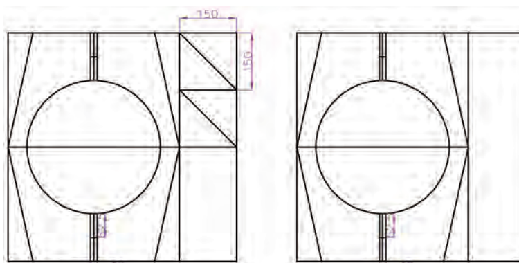
شکل ۳۸- خط‌کشی شکاف‌ها
