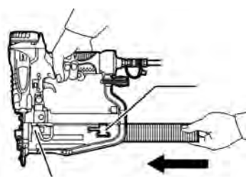
شکل ۱۰۲- بارگذاری منگنه
