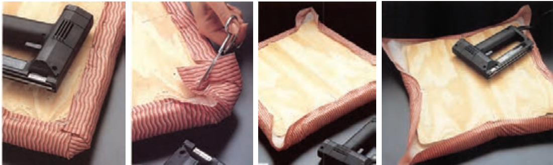
شکل ۸۸- ثابت کردن پارچه شکل ۸۹- کوبیدن پارچه شکل ۹۰- قیچی کردن گوشه ها شکل ۹۱- گوشه های منگنه خورده
