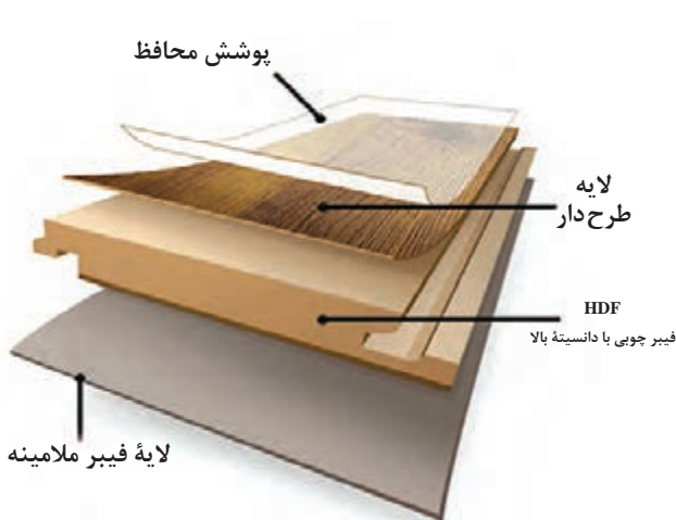
شکل ۱۲- انواع کف‌سازی باصفحات روکش‌دار
