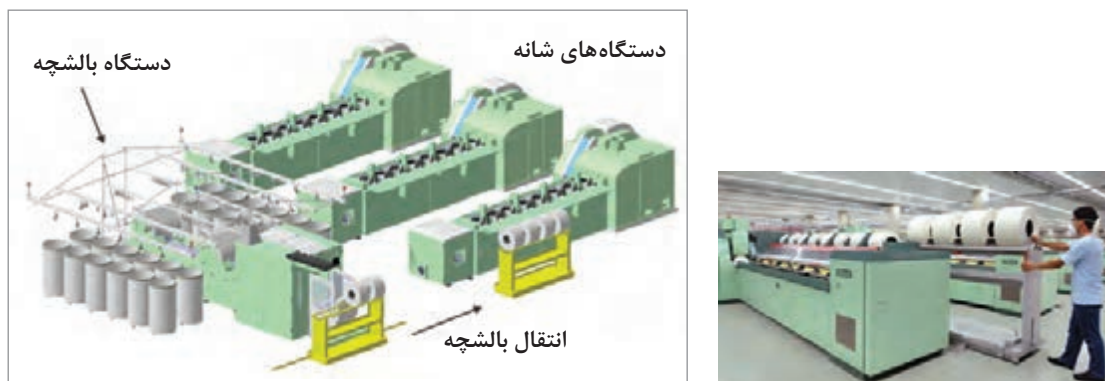
شکل ۲۶- انتقال قفسه بالشچه به قسمت تغذیه شانه
