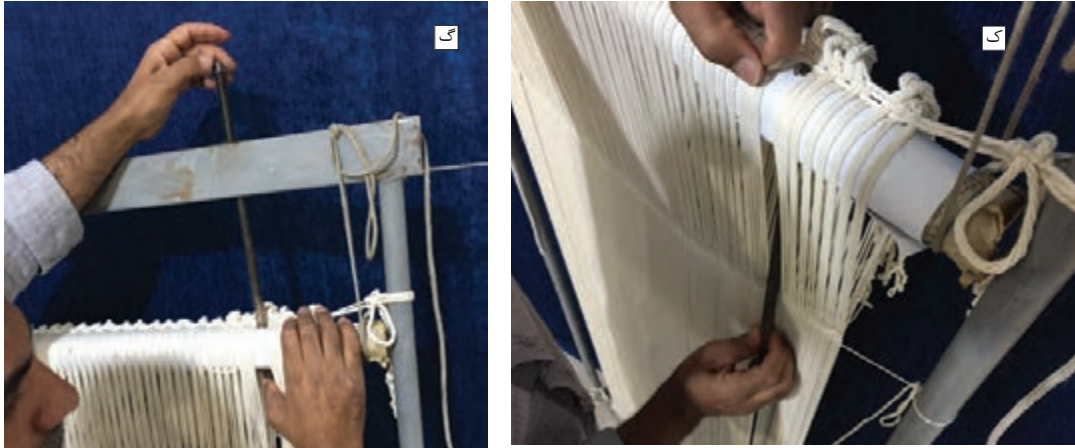
شکل ۱۳-۳- گره زدن دسته‌های چله بر روی سردار و تنظیم آنها
