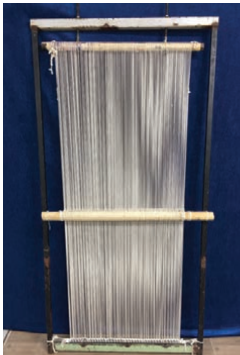
شکل ۱۱-۱- دار قالی فنکدار
