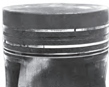
شکل ۴-۱۰۱- چسبندگی رینگ
