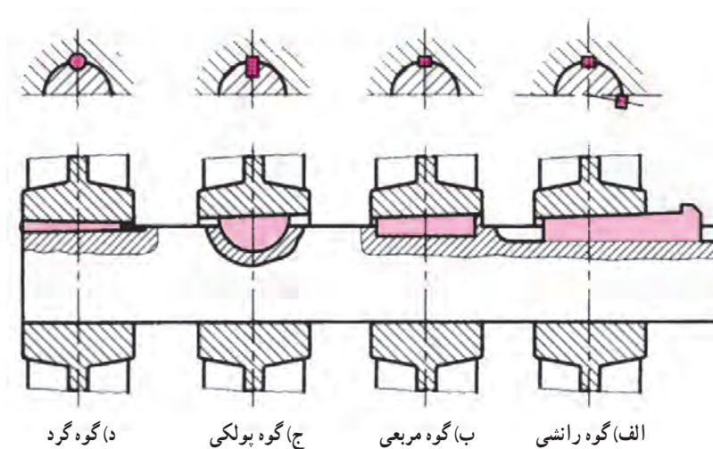
شکل ۳-۲۲- انواع گوه
