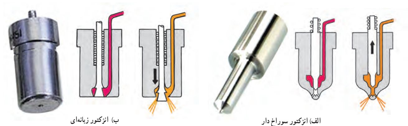
شکل ۱۷-۴- انواع انژکتور
