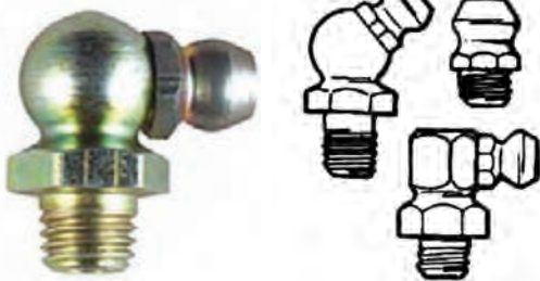
شکل ۵۴-۷- انواع گریس خور از نظر زاویه قرار گرفته
