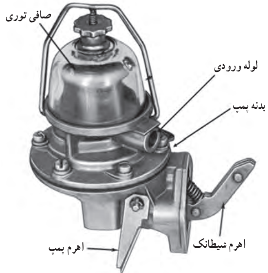
شکل ۴-۴ - اجزای پمپ مقدماتی دیافراگمی
