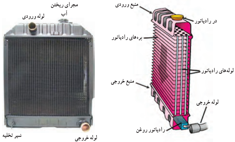
شکل ۳-۳- اجزای رادیاتور
