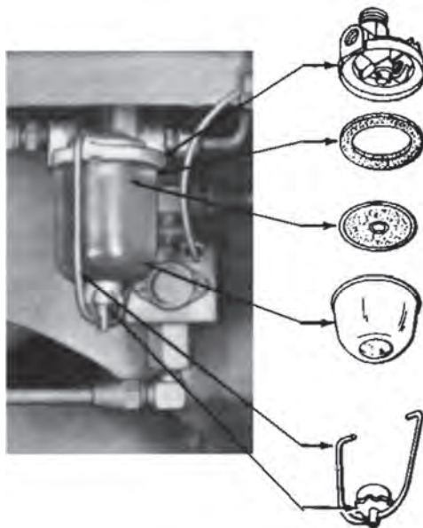
شکل ۱۰-۴- پایاله رسوب گیر
