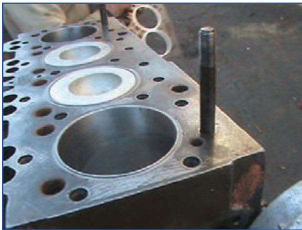
شکل ۵۳-۴- کنترل تمیز بودن سطح سرسیلندر و باز بودن مجاری
