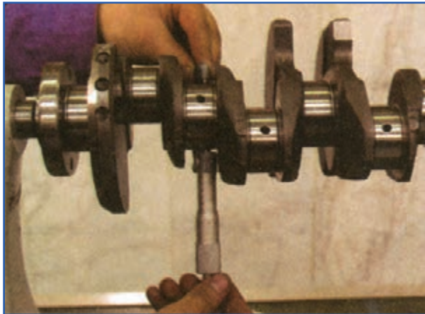
شکل ۱۶۲-۴- اندازه‌گیری قطر محورهای میل‌لنگ
