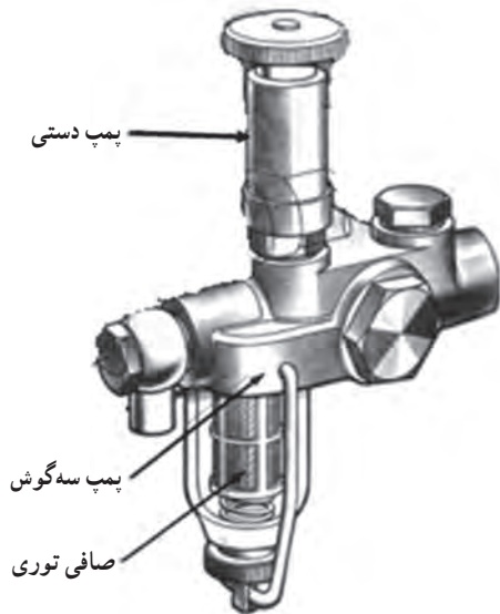
شکل ۴-۵ - اجزای پمپ مقدماتی پیستونی
