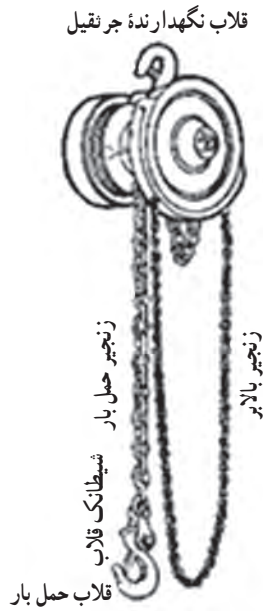
ب) اجزاء جرثقیل سقفی
