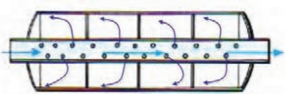
شکل ۲۴-۵- صدا خفه‌کن یکسره
