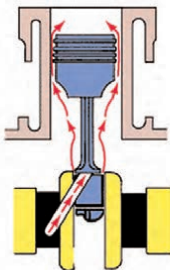
شکل ۴-۷- روغن کاری یاتاقان متحرک و رینگ‌ها
