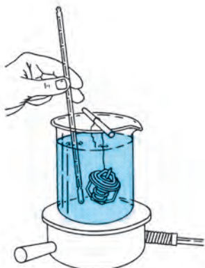
شکل ۲۲-۳- آزمایش ترموستات
