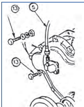
شکل ۴-۵۷- خارج کردن پولی میل‌لنگ
