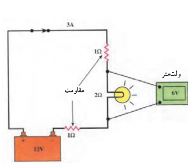
شکل ۷۵-۶ ایجاد مقاومت در مدار به صورت سری باعث کاهش ولتاژ در مدار می‌گردد.
