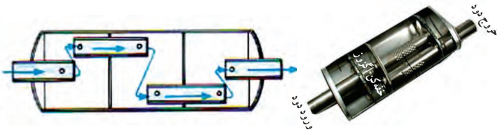
شکل ۲۵-۵- خفه‌کن معکوس
