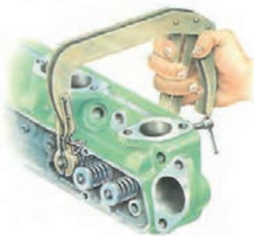
شکل ۱۷-۴- نحوه قرار دادن سوپاپ باز کن روی سوپاپ‌ها
