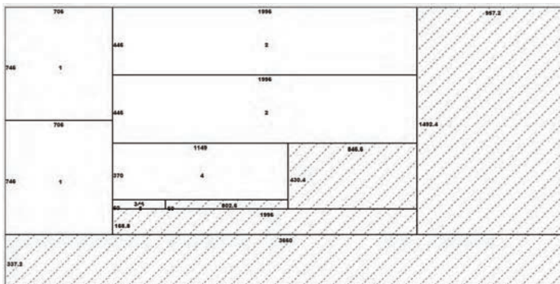
شکل ۲۶- نقشه چیدمان میز کنفرانس در ورق رنگی ۱ به ابعاد 366 \times 183 سانتی‌متر
