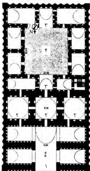
پلان
