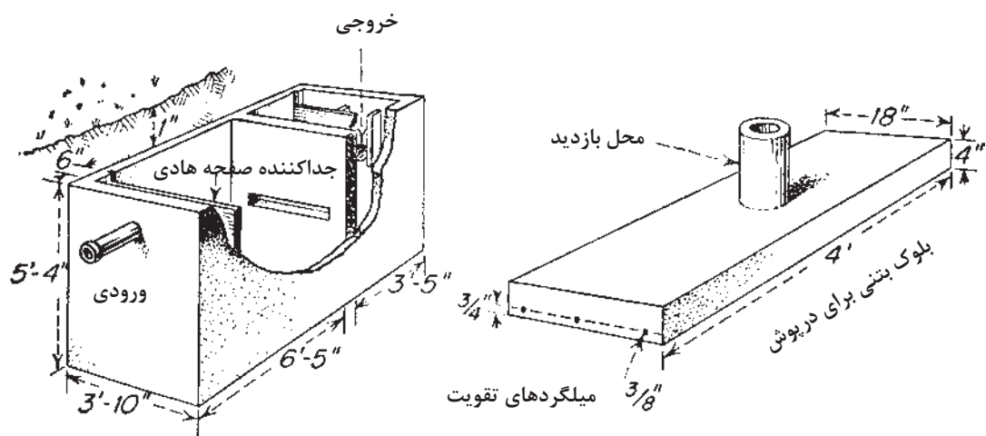
شکل ۴-۴۴- سپتیک تانک
