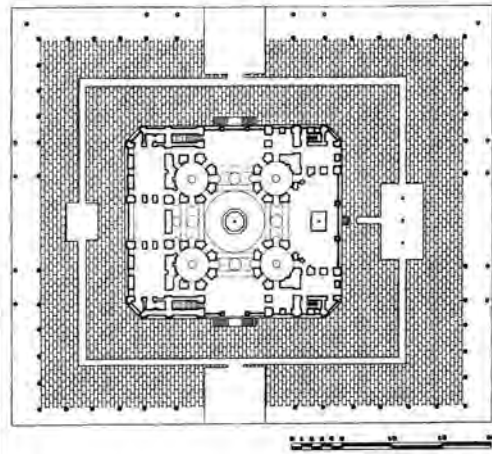
سایت پلان
