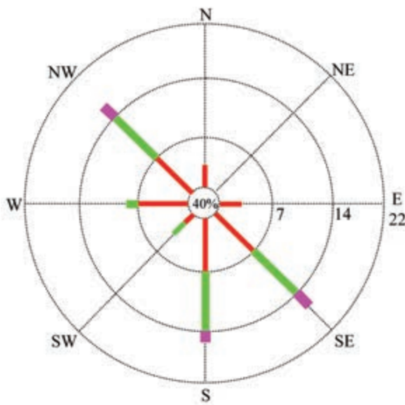
شکل ۲-۳- گلباد ایستگاه کرج در تابستان
