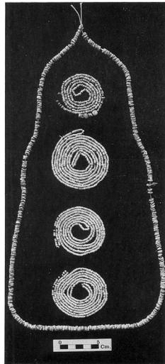
شکل ۱-۱۰-۱ تعدادی از آثار کشف شده از محوطه ازبکی
