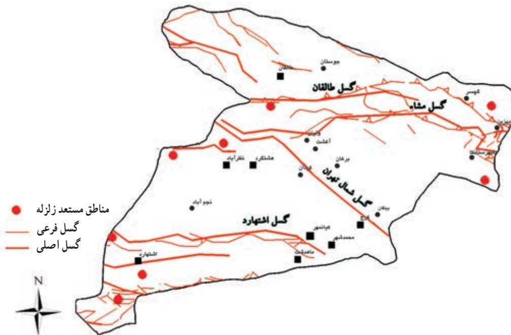
شکل ۱-۵- نقشهٔ پراکندگی گسل‌های اصلی استان
