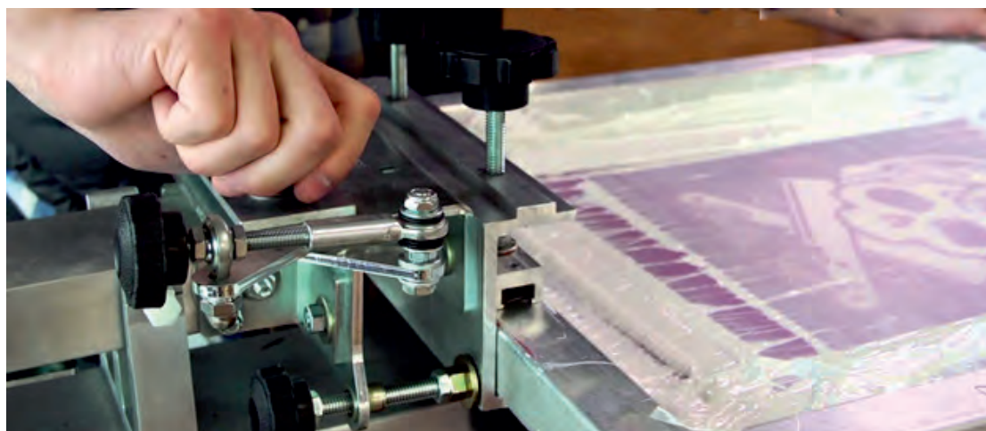
(شکل ۴-۴) گونیا کردن طولی و عرضی شابلون
