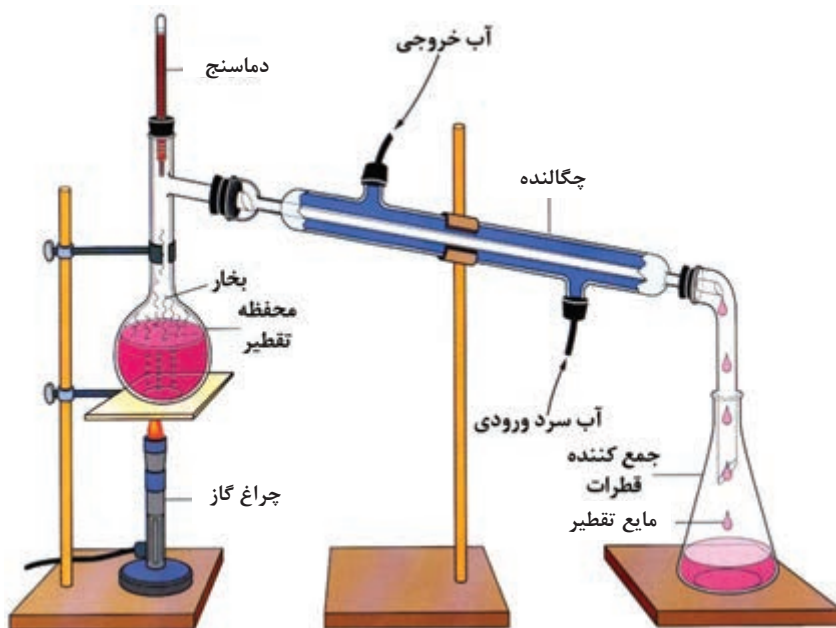
شکل ۶-۴- دستگاه تقطیر
