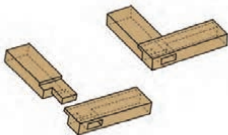
شکل ۱۲- تصویر سه بعدی از اتصال کم و زبانه کوله‌دار
