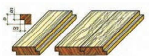
شکل ۳۱- اتصال عرضی نیم ونیم
