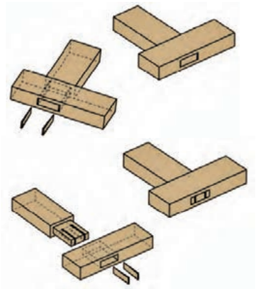
شکل ۱۹- اتصال کم و زبانه با دو شیار روی زبانه و دو گوه چوبی که درون شیارها قرار می‌گیرند.
