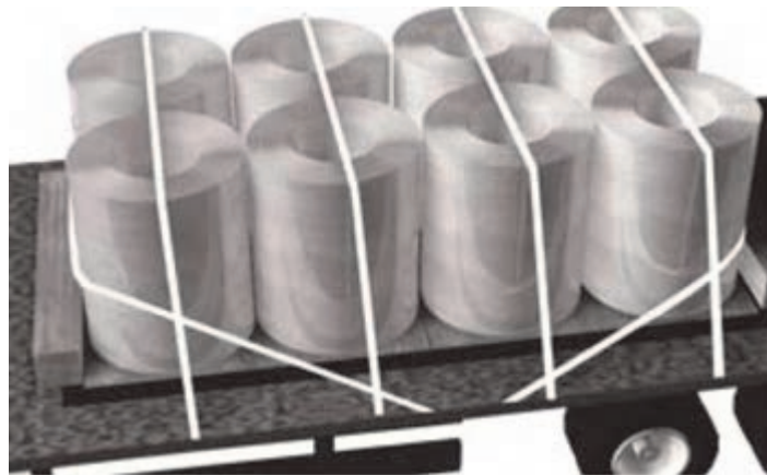
شکل ۳۴- نحوه کاهش بندها در مه‌ار بارهای استوانه‌ای
