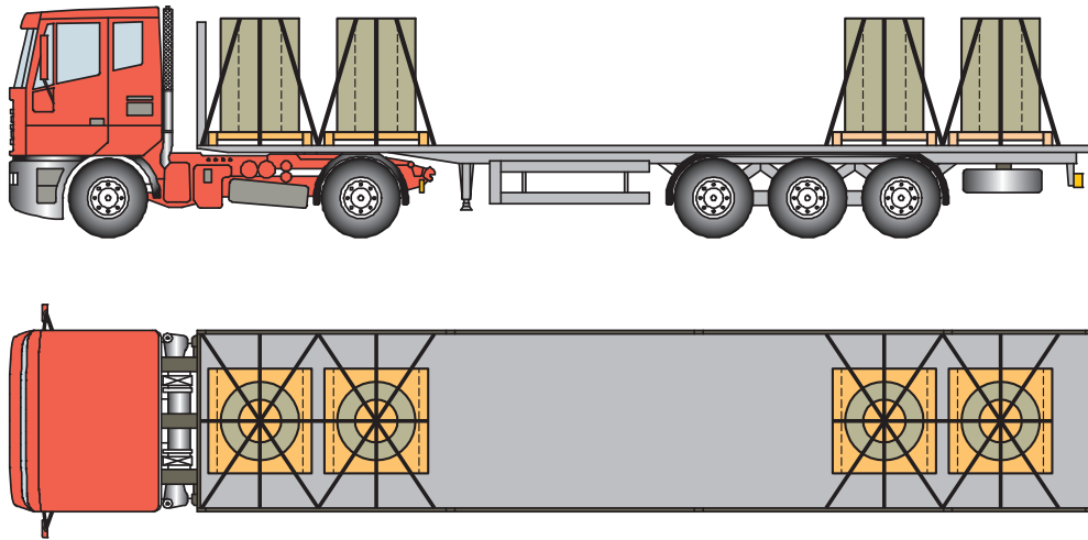
شکل ۳۳- نحوه مه‌ار رول‌های عمودی
