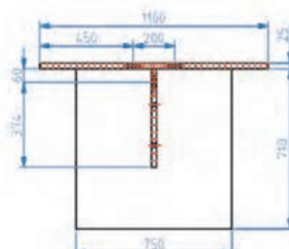
A-A (1:20)
