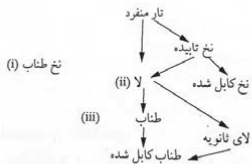
نمودار ۱ - ساختار کلی تولید انواع طناب‌های تابیده
