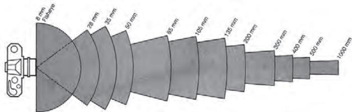
تصویر ۸-۶- دیاگرام زاویه دید لنزهای مختلف
