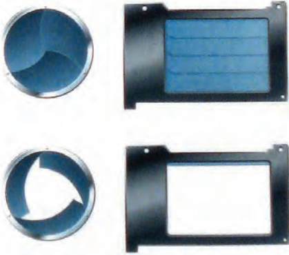
تصویر ۲-۲- شاترهای مرکزی و کانونی در ۲ حالت باز و بسته
