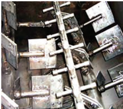
تصویر ۱۴-۵- مخلوط‌کن مجهز به همزن
