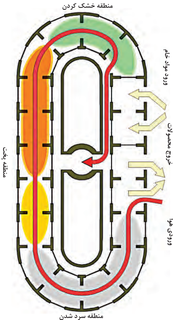
شکل ۱۳- کوره هوفمن
