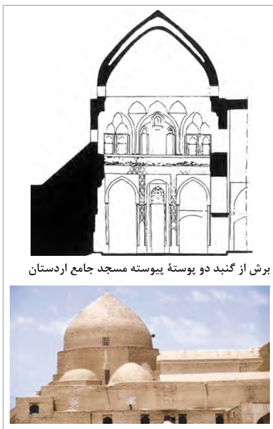
شکل ۱-۱۶۷- مسجد جامع اردستان و گنبد دوپوسته آن
