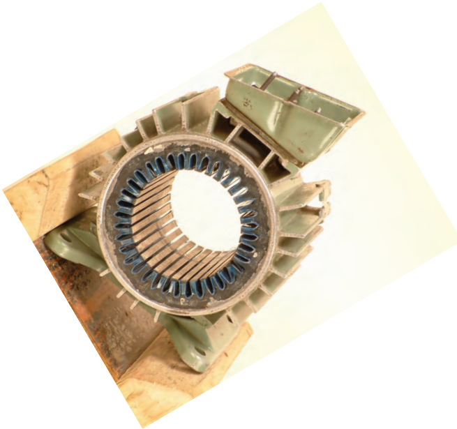
شکل ۱۲-۲- پوسته موتور سه فاز ۳۶ شیار
