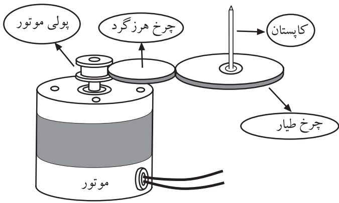
شکل ۳-۷- سیستم چرخ‌هرزگرد
