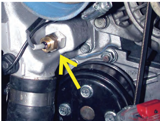
شکل ۴-۱- محل نصب سنسور آب
