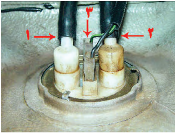
شکل ۱-۱۶- قسمت خارجی شناور
