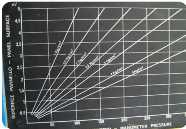
شکل ۸۱-۵- دیگرام یا منحنی رابطه بین سطح و فشار در یک پرس روغنی
