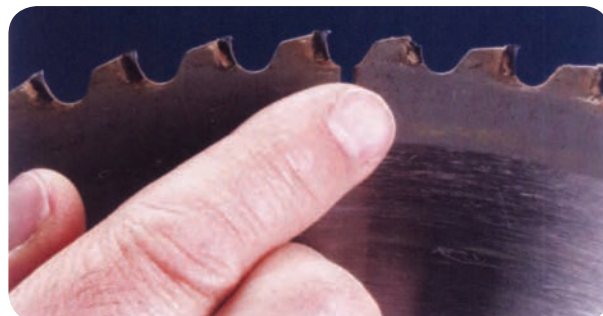
شکل ۴۲-۵- دندان‌های اره شکسته یا کند شده
