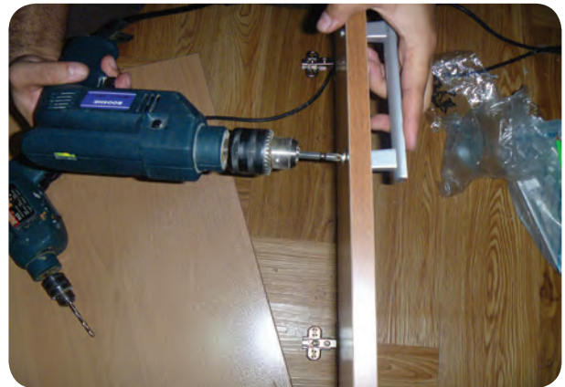
شکل ۱۷۸-۵- نصب دستگیره
