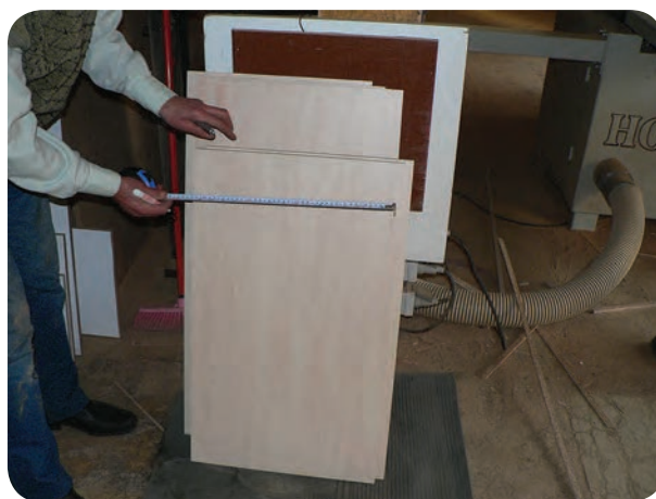
شکل ۱۱۶-۵- کنترل اندازه قطعات آماده شده
