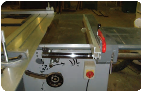
شکل ۵-۵۳- فرمان تنظیم ارتفاع برش
