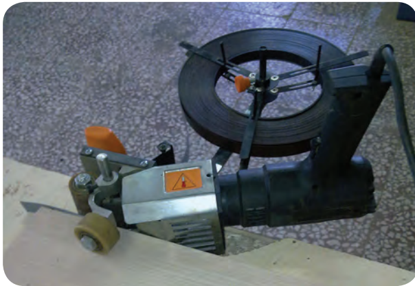
شکل ۴-۲۲ - نحوه نوار کردن قطعه کار به کمک سشوار نصب شده روی میز
