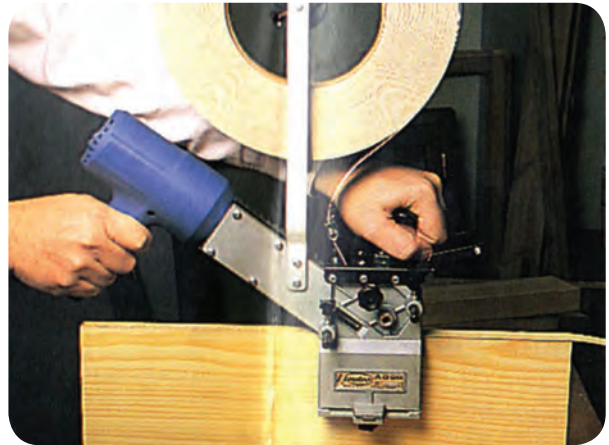
شکل ۴-۱۹ - نحوه نوار کردن با سشوار
