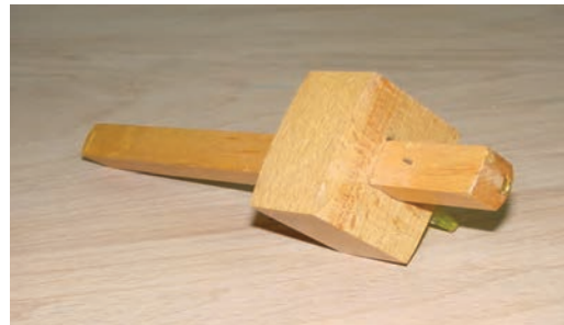
خط‌کش تیره‌دار
