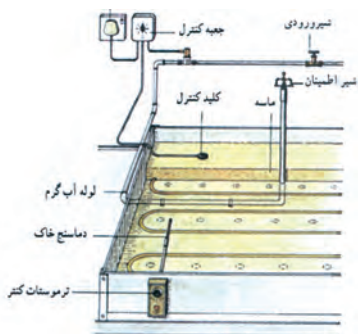
شکل ۱۳- نوعی سیستم گرمایشی
