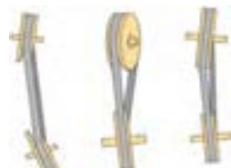
شکل ۱۶-۲- غیرهم‌راستایی محوری و زاویه‌ای پولی‌ها
