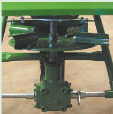
صفحه دوار
