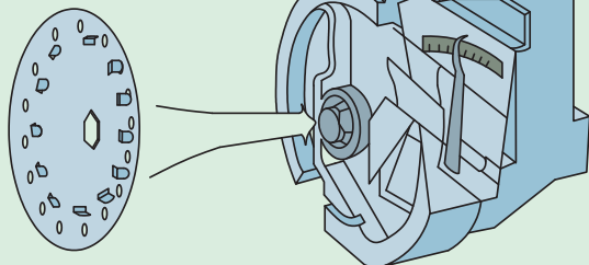
شکل ۴۷-۳. جهت بستن صفحه موزع نیوماتیک
