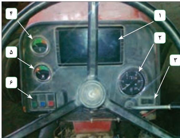
شکل ۳- وسایل اندازه‌گیری و هشداردهنده تراکتور
