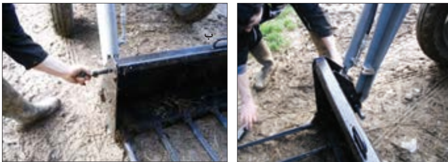
(الف) (ب) شکل ۳۱-۴-۱ اتصال باکت‌ها به بیل
