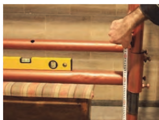
شکل ۱۹ و ۲۰- بستن اجزاء دستگاه با رعایت صحیح فواصل و موازی با افق
