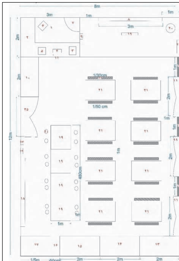
شکل ۱۳-۱. پلان کارگاه جاجیم بافی
