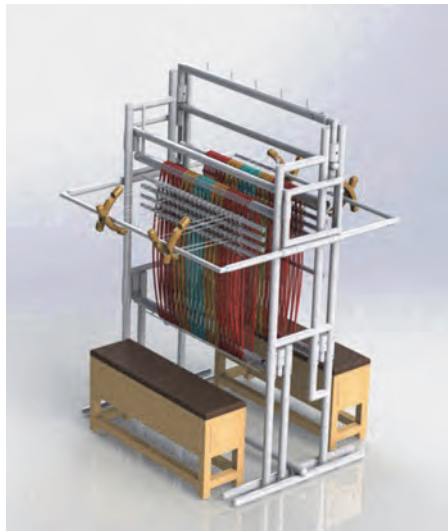
شکل ۲۱- دستگاه بافت و نیمکت
