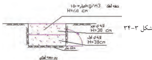
شکل ۳-۳۳ پی شفته آهکی
