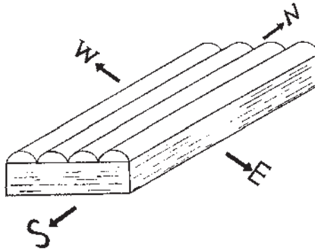
شکل ۱۰-۲ - جهت شمالی جنوبی مناسب گلخانه ای چند واحدی
