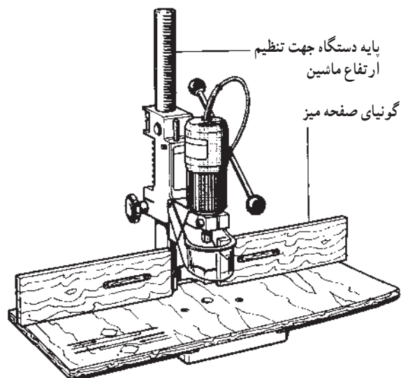
شکل ۸-۵۱- استقرار فرز روی صفحه میز
