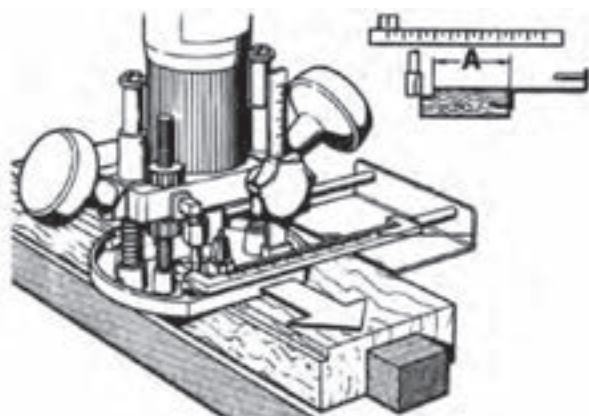
شکل ۱۲-۸- با قراردادن گونیا در کنار قطعه کار، فاصله محل ابزار تا لبه‌ی کار مشخص می‌شود.
