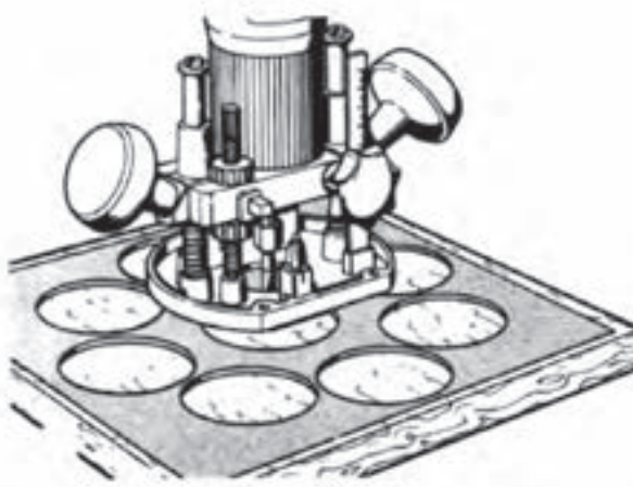
شکل ۸-۲۶- طرز تنظیم ماشین فرز و تکیه‌دادن آن به پایه راهنما جهت یخ‌زدن لبه‌ی دایره روی صفحات
