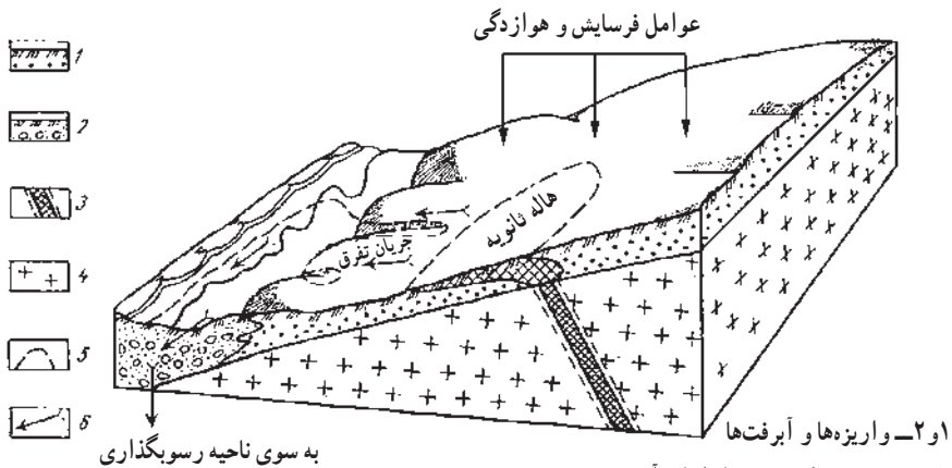
شکل ۱۳-۲- هاله ثانویه و گسترش آن ۱ و ۲- واریزه‌ها و آبرفت‌ها ۳- توده معدنی اصلی و هاله اولیه آن ۴- سنگ‌های دورنگیر ۵- محدوده آنومالی ۶- جهت حرکت مواد [۱۵].
