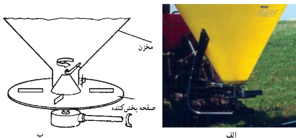
شکل ۴۰-۱- پخش‌کننده صفحه‌ای
