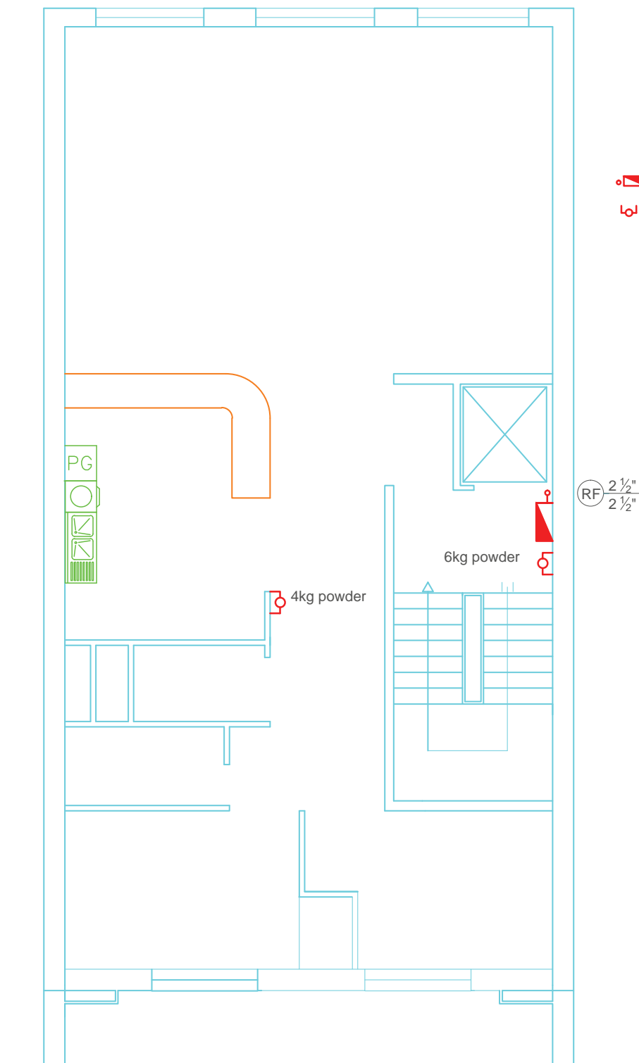
شکل ۲-۴-ب- پلان لوله کشی آب آتش نشانی طبقات - مقیاس ۱/۱۰۰
