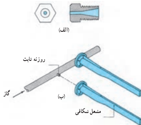
الف) روزنه قابل تعویض
