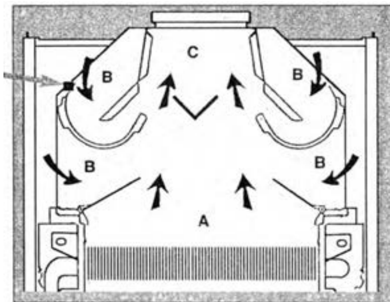
A: محصولات احتراق متصاعد شده از محفظه احتراق و مبدل اولیه B: ورود هوای تازه C: دودکش به قطر ۱۲۵ یا ۱۳۹ میلی متر D: محل قرارگیری ترموستات دود
