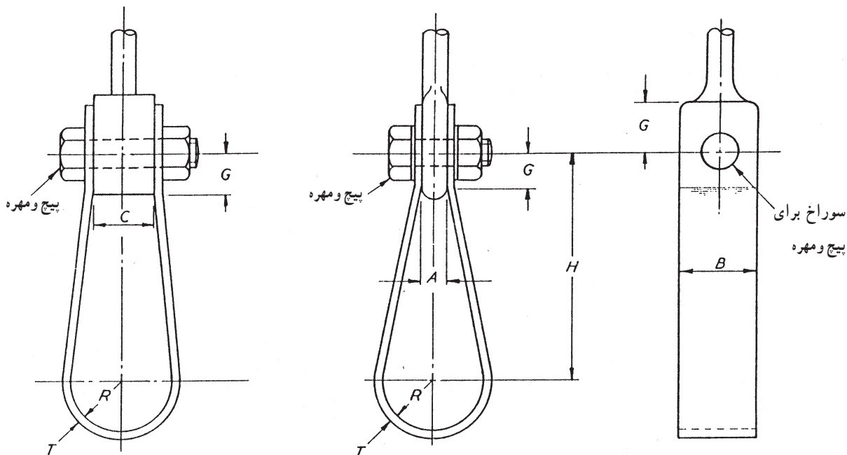
شکل ۱۱-۲- نوعی بست آویز تسمه‌ای یک تکه
