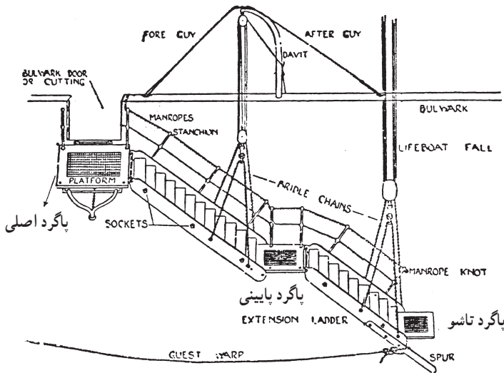
شکل ۶۱-۵. پله تشریفاتی
