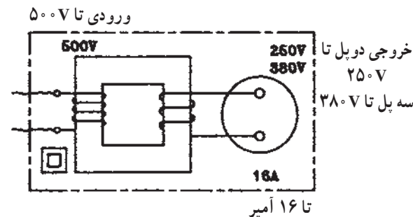
شکل ۸-۱۰ ترانس ایزوله
