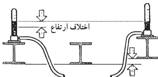
شکل ۱۳-۳ شیلنگ تراز
