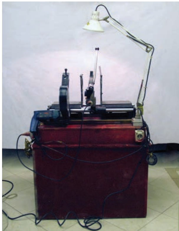
شکل ۲-۳۷- دستگاه جوش لوله و فیتینگ پلی اتیلن
