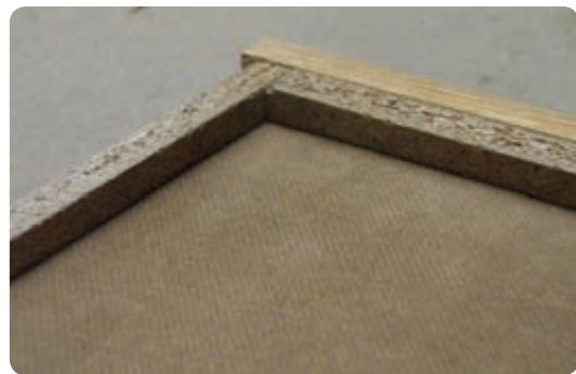
شکل ۶-۱۰۳ کف جعبه در کنشکاف بدنه جعبه و در جعبه
