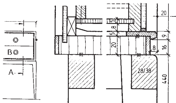
شکل ۴-۷۸- دتایل یا برش A-A
