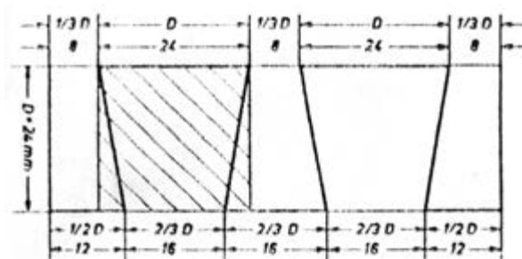
شکل ۴-۱۰۲ نسبت‌های ترسیم شده اتصال دم چلچله ساده
