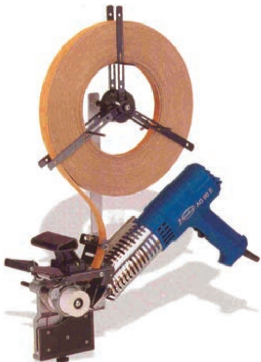
شکل ۱۴۸- نوار لبه‌چسبان سشواری
