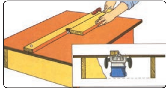
شکل ۶۲-۲ بکارگیری اورفرز در حالت میزی
