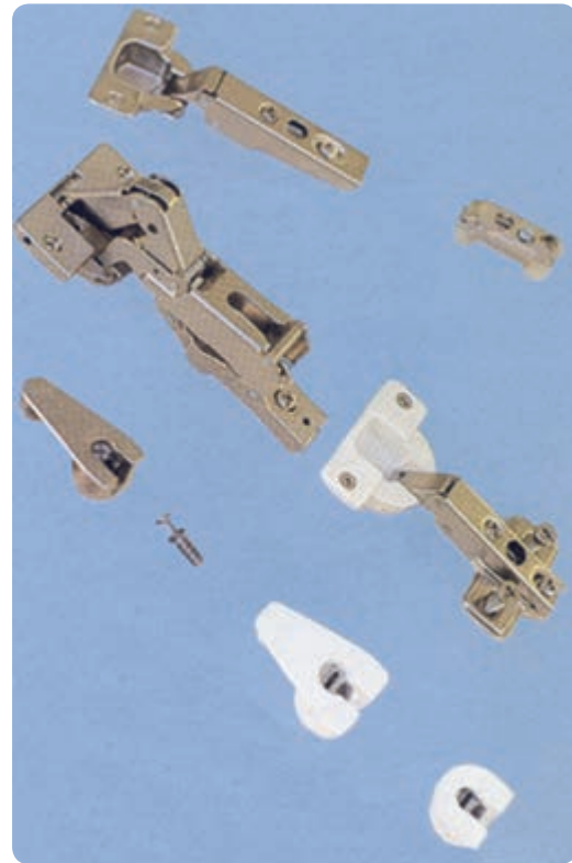
شکل ۲-۱۲۱ لولای فنردار اتومات کابینت (لولازن)
