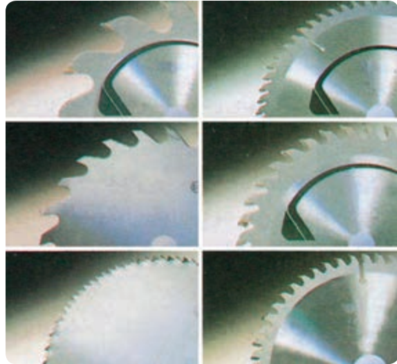
شکل ۲-۳۵ چند نمونه از تیغه‌های گرد (مجموعه‌ای) جهت برش مواد چوبی و غیر چوبی
