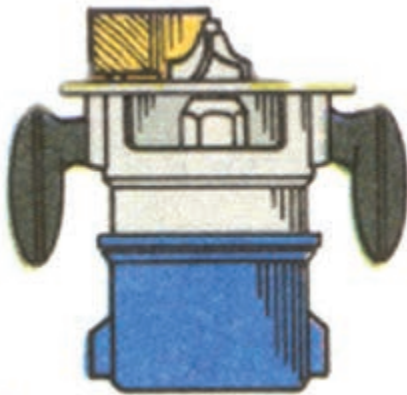
شکل ۲-۴۳ تنظیم ارتفاع تیغه اور فرز
