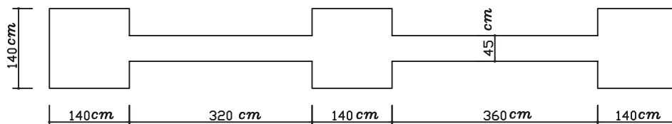
پلان فونداسیون
