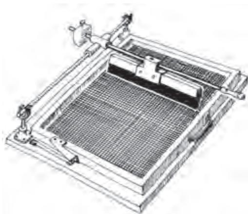
تصویر ۱۲۷- نوعی دستگاه برای چاپ شابلونی
