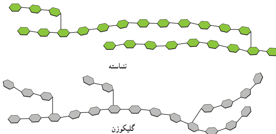
شکل ۲-۲- مولکولهای نشاسته و گلیکوژن
