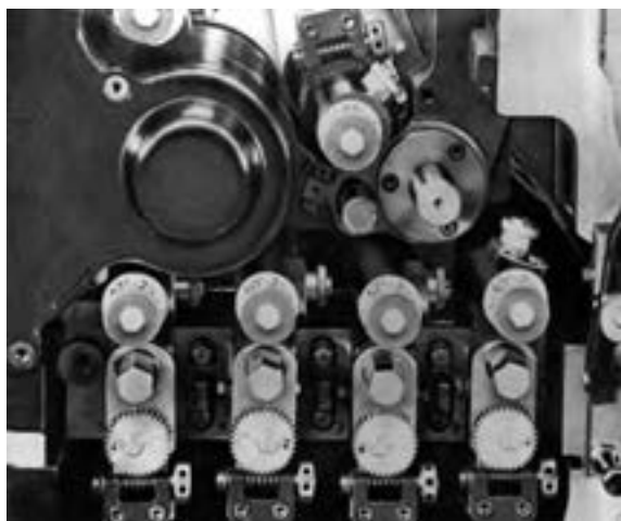
شکل ۱۴-۴- تنظیم ارتفاع نورد‌های منتقل‌کننده رنگ به وسیله چرخ‌دنده‌های خارج از مرکز
