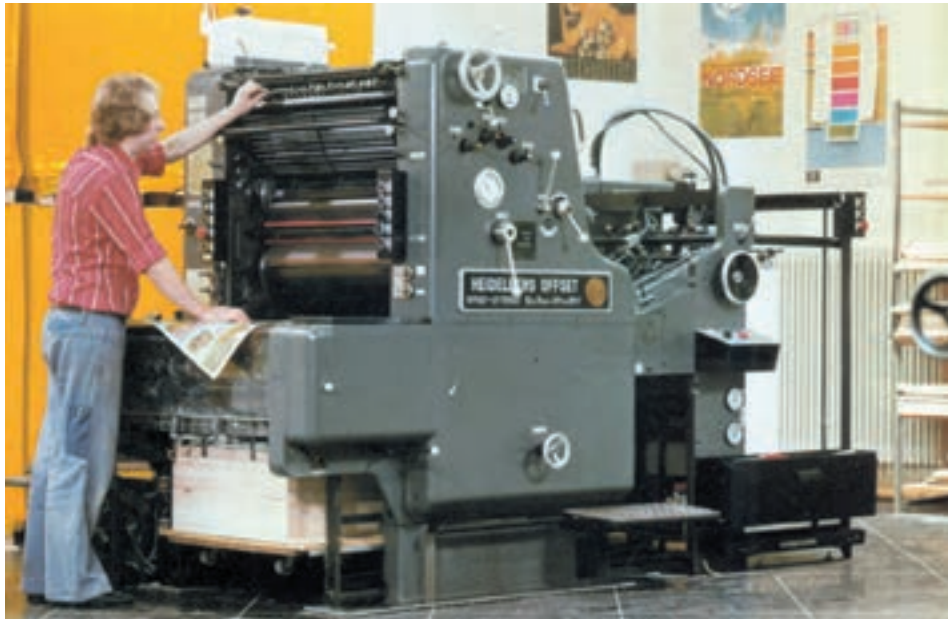
شکل ۱۵-۲- ماشین روتاسیون ورقی یک رنگ آفست یا لترست (برجسته)
